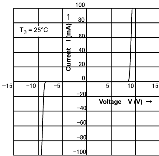
Fig. 8.1 I - V
