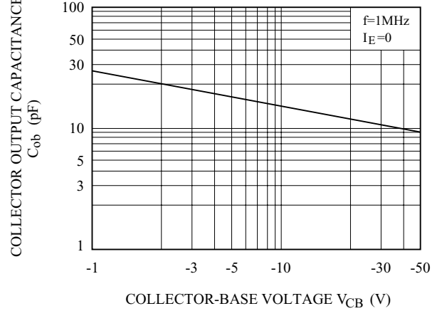
C_{ob} - V_{CB}
