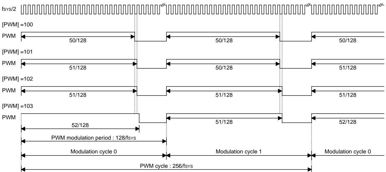
(7+1)位模式 PWM
