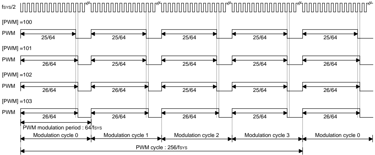
(6+2)位模式 PWM
