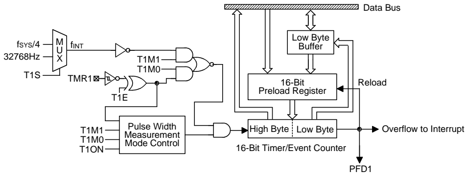
定时/计数器 1
