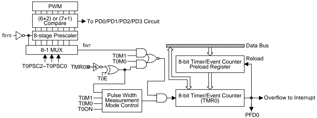
定时/计数器 0
