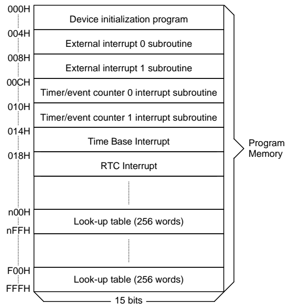
程序存储器
