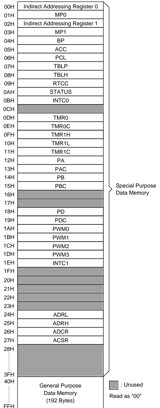
数据存储器
