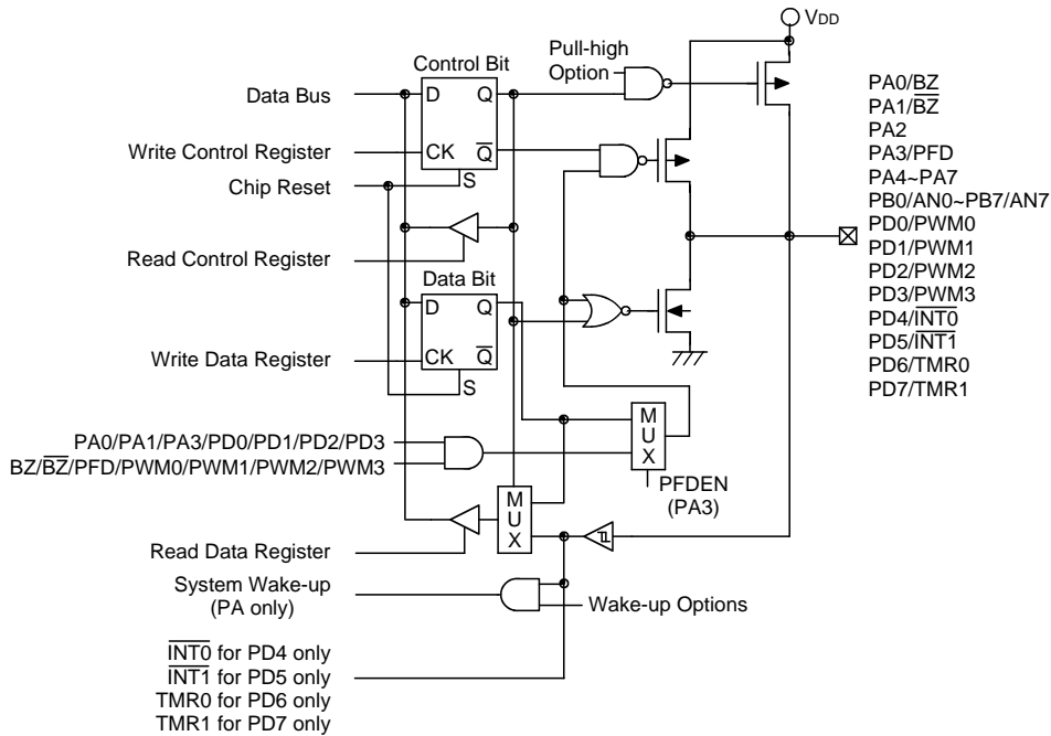
输入/输出口
