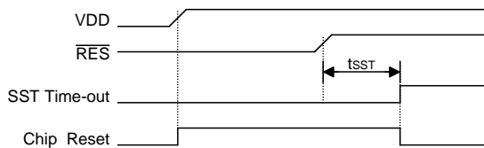
复位时序图
