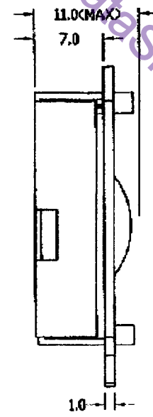
DETAIL A:
