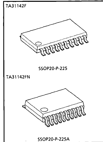
Weight SSOP20-P-225 : 0.18g (Typ.) SSOP20-P-225A : 0.09g (Typ.)
