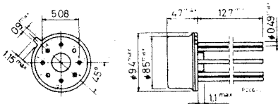
TO-99
