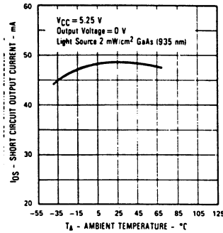
OPB900L, OPB902L, OPB910L, OPB912L Short Circuit Output Current vs Ambient Temperature
