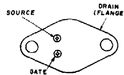
JEDEC TO-204AA
