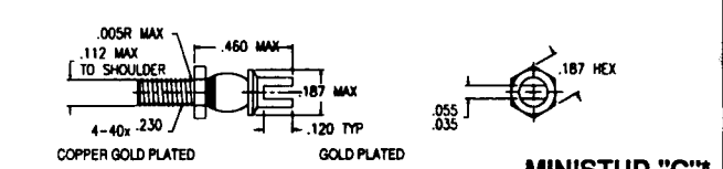
MINISTUD "C"
