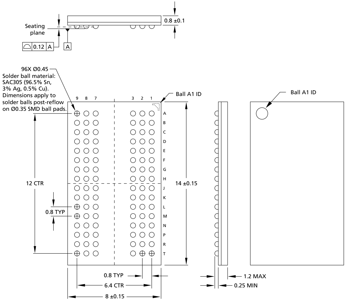
Figure 6: 96-Ball FBGA – x16; Die Rev. K (JT)
