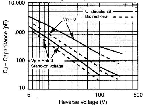
Fig. 6 – Capacitance
