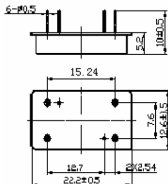
外壳外形结构图
