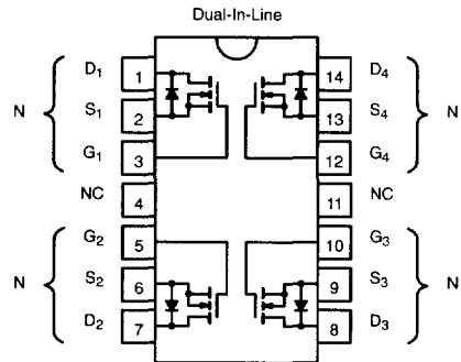
Top View Sidebraze: VQ1006P
