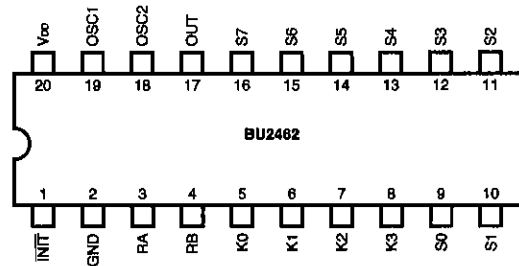
BU2462 pin layout
