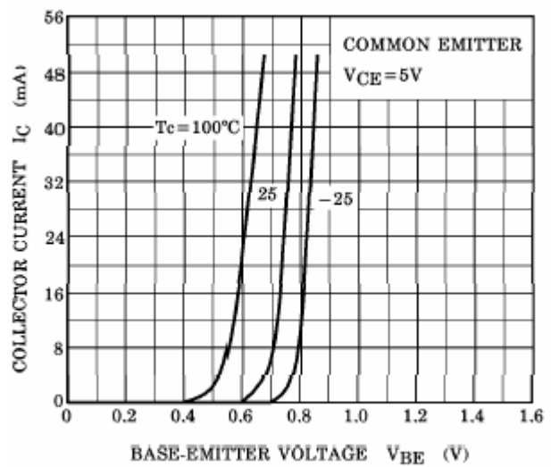
Fig.4 I_C - V_{BE}
