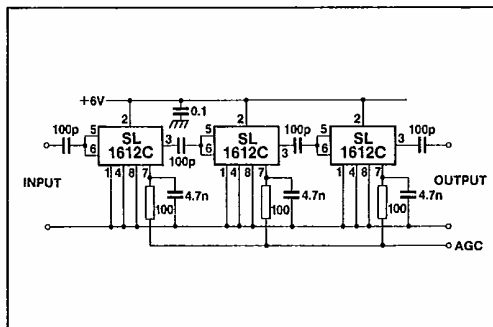
Fig. 9 IF amplifier using SL1612
