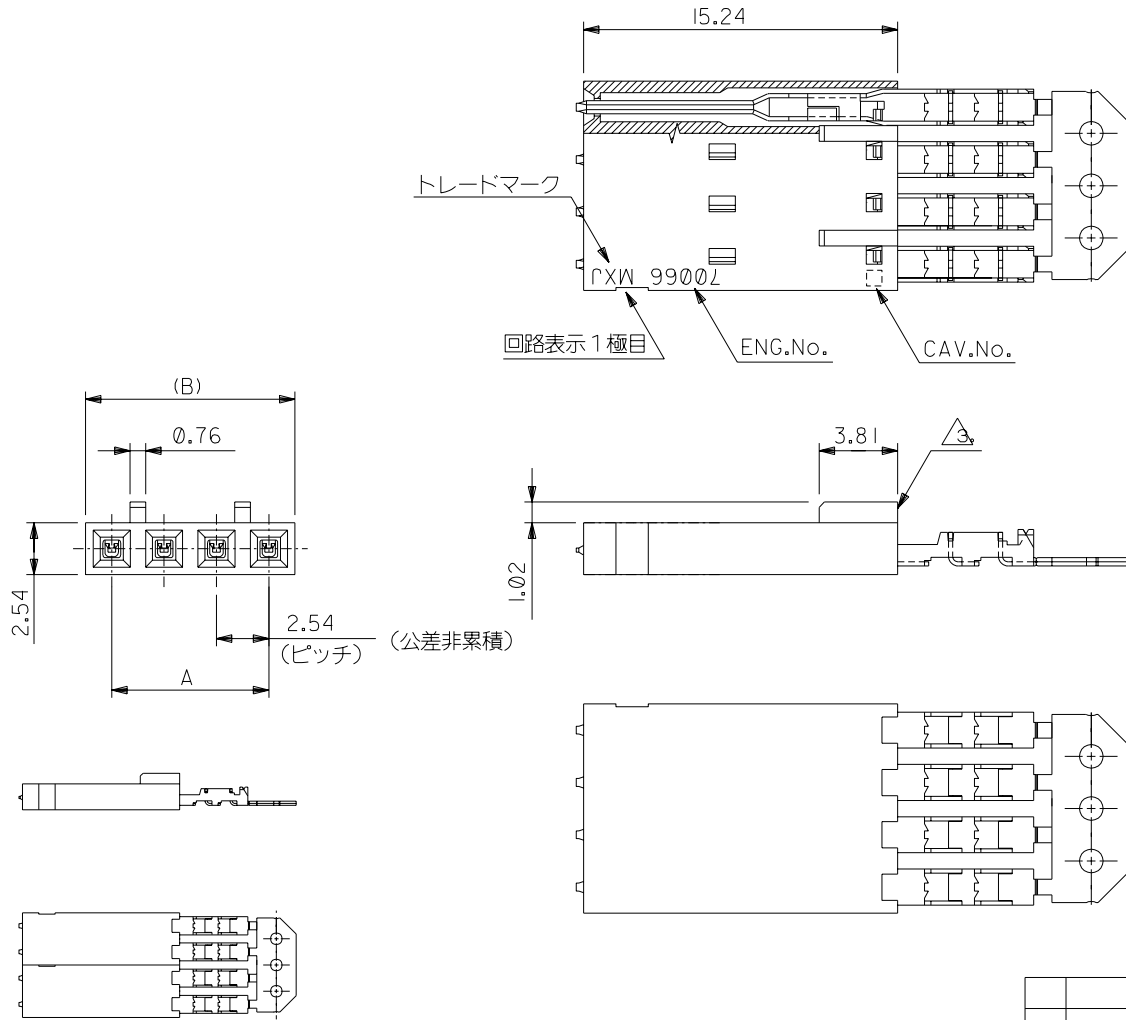
2 極の場合 (SCALE:2-1)
