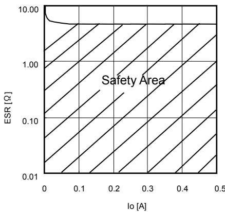
Fig.17 ESR condenser
