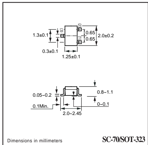
SC-70/SOT-323
