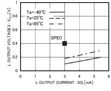
Fig.13 'L' Output Voltage3 V OL3 -I OL (V CC3 =3.0V) (SDA3)
