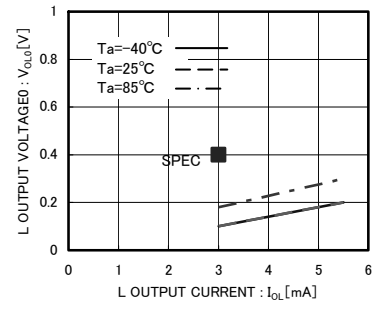
Fig.10 'L' Output Voltage0 V OL0 -I OL (V CC0 =3.0V)
