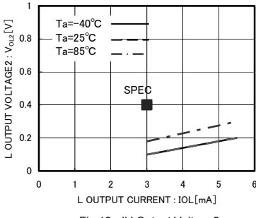
Fig.12 'L' Output Voltage2 V OL2 -I OL (V CC2 =3.0V) (SDA2)
