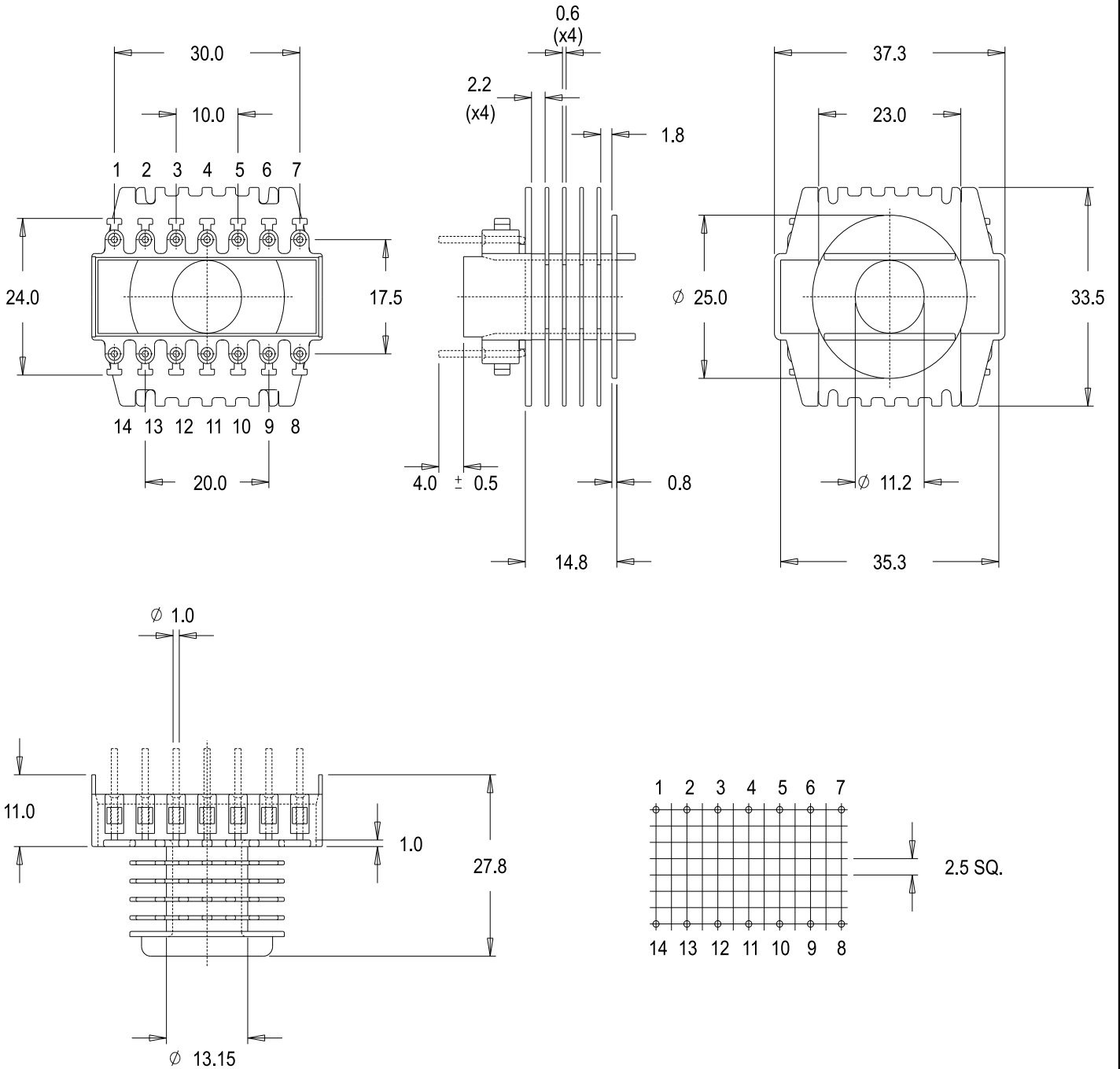
ETD-34-K-V-5-CHAMBER
