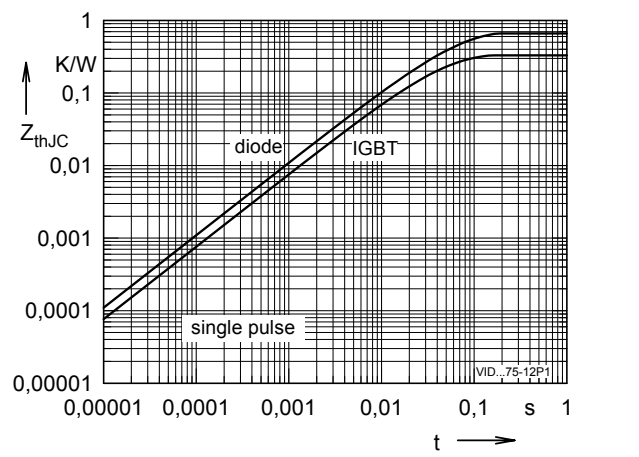
Fig. 12 Typ. transient thermal impedance RBSOA
