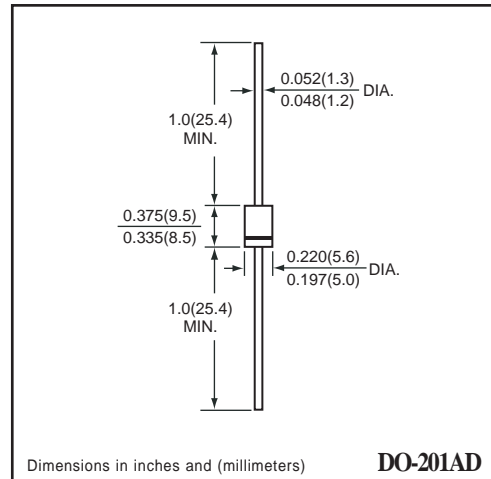
DO-201AD
