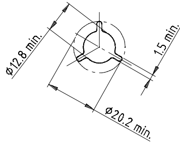
Reel hub 2:1
