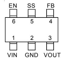
SOT-23-6 / TSOT-23-6 / SC-70-6
