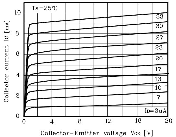
Fig. 2 I_C - V_{CE}
