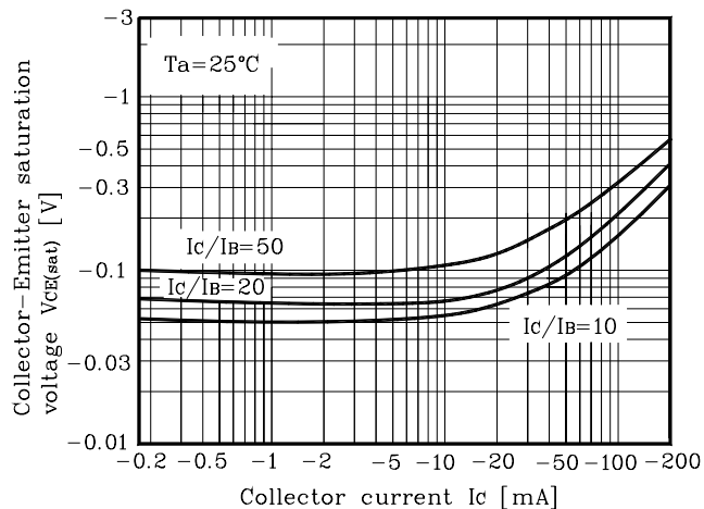
Fig. 4 V_{CE(sat)}-I_C
