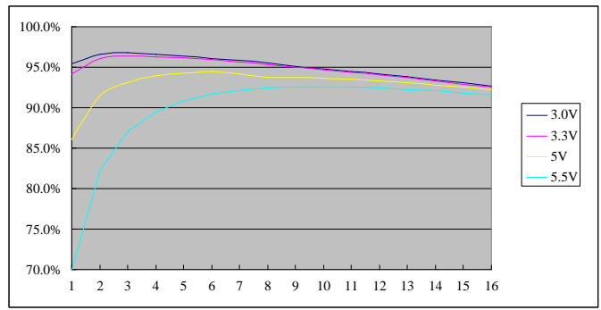
Vo=2.5 V
