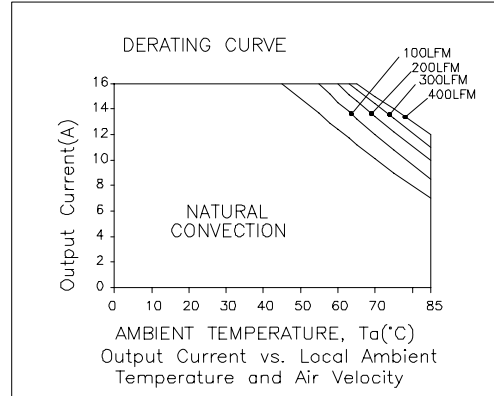
Vin=5.0 V, Vo=1.5 V or 1.8 V
