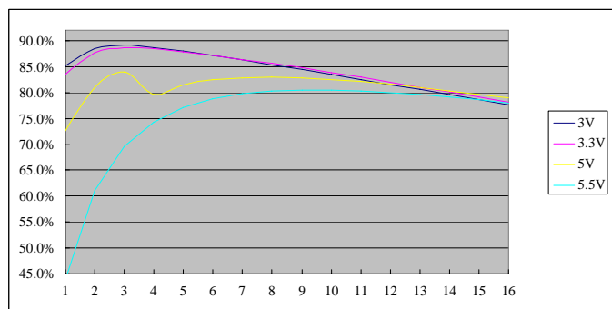
Vo=0.7525 V
