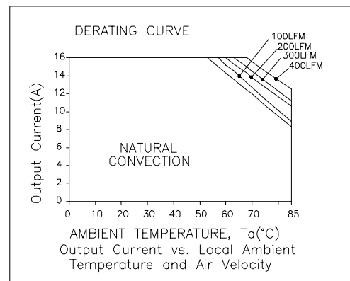
Vin=3.3 V, Vo=1.5 V or 1.8 V
