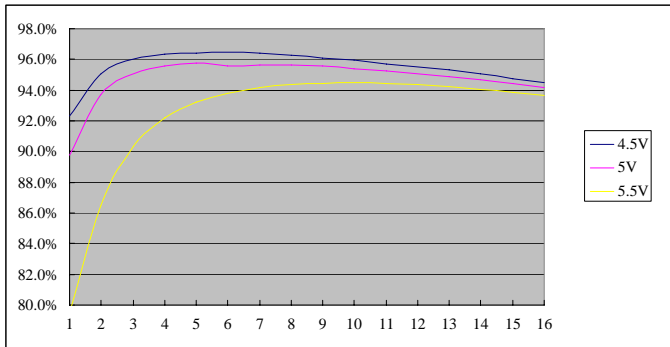
Vo=3.3 V
