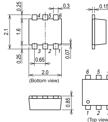
外形図 2173A (unit : mm)
