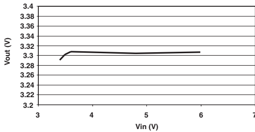
Vout Vs. Vin* Iout = 0.1A
