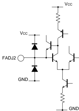
4pin (44pin)
