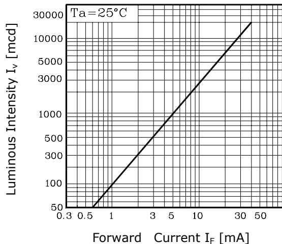
Fig. 2 I_V - I_F
