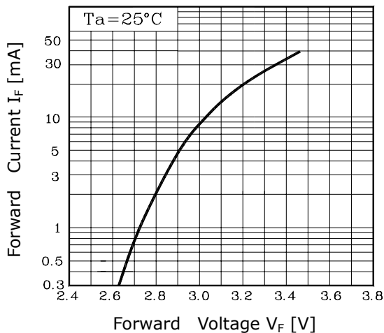
Fig. 1 I_F - V_F
