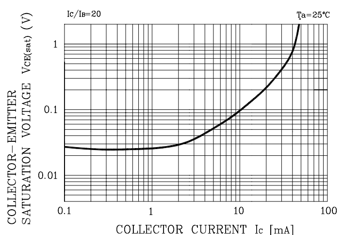
Fig. 2 V_{CE(SAT)} - I_C
