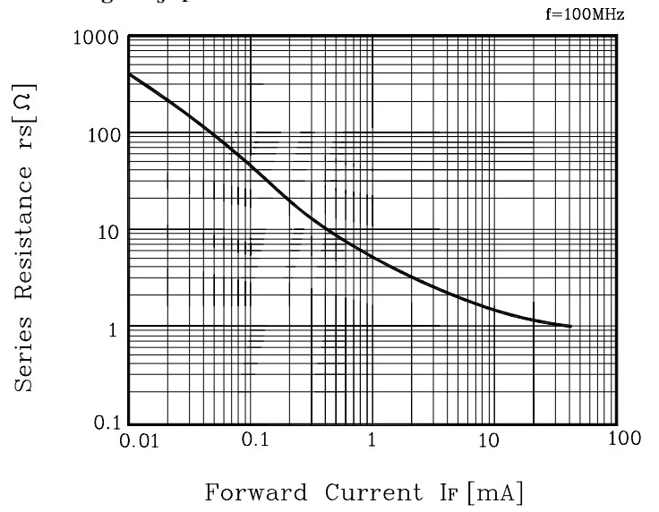
Fig. 2 r_s - I_F
