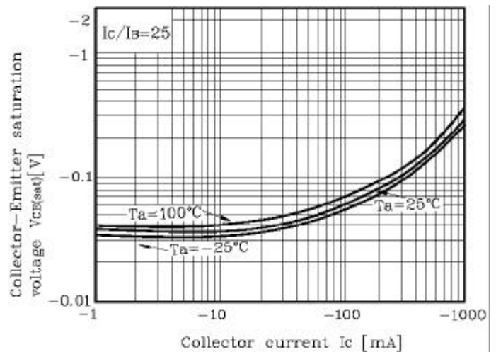
Fig 5. V_{CE(sat)} - I_C
