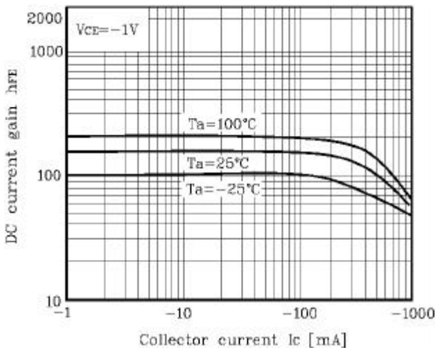
Fig 5. h_{FE} - I_C
