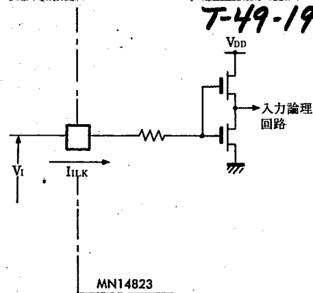
Fig. 2 入力回路(Fig. 4 参照)
