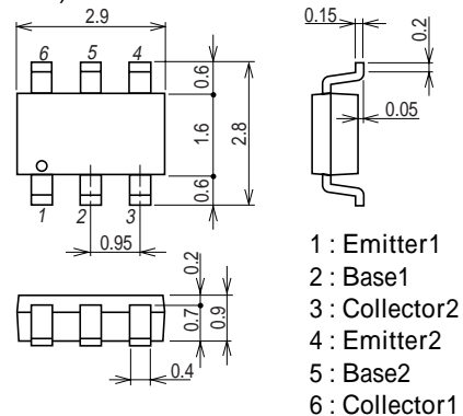
外形図 2187
