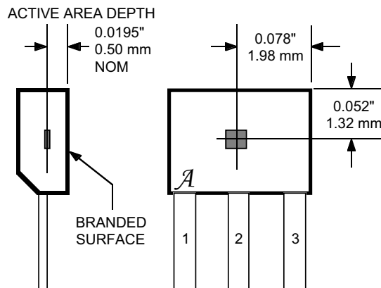
Dwg. MH-011-13
